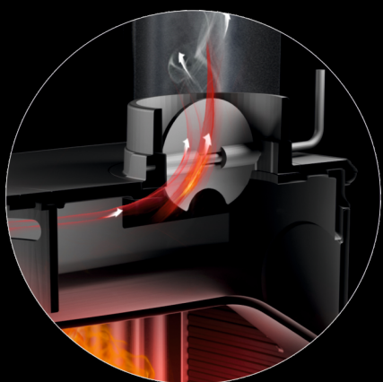
Поворотный шибер
